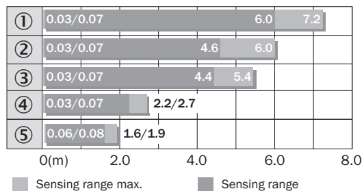
触发感应距离图表 GL6
