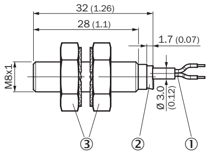
尺寸图 IMB08 短版, 电缆, 齐平
